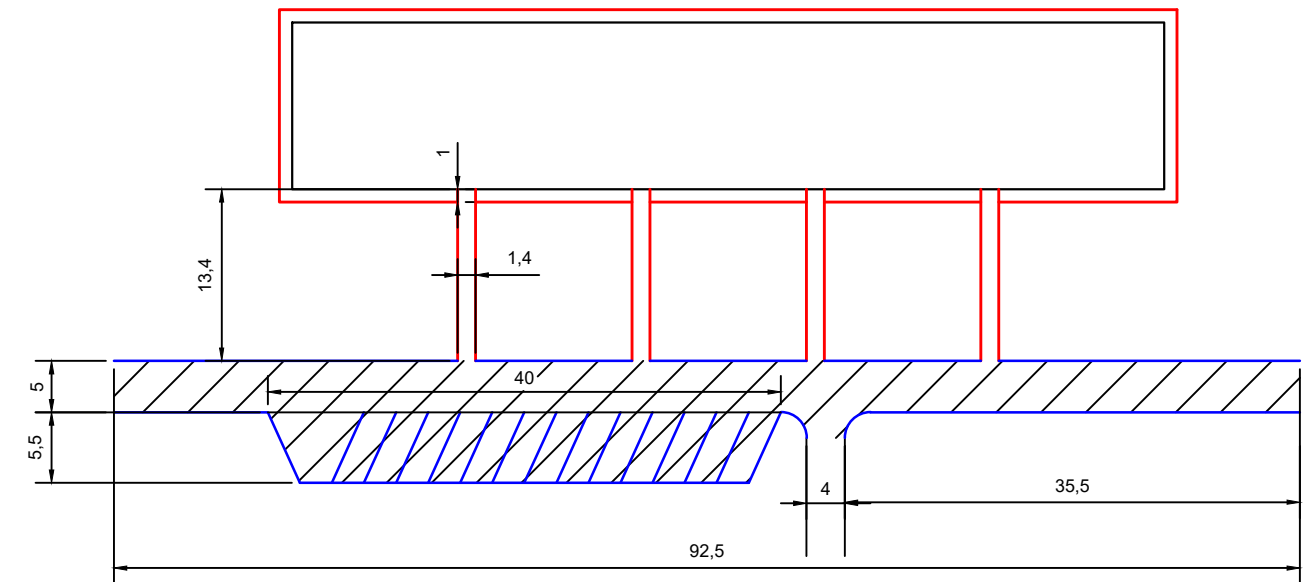
Генеральный план благоустройства дворовой территории п. Тайжина, ул. Коммунистическая, 22 (М1:500)
